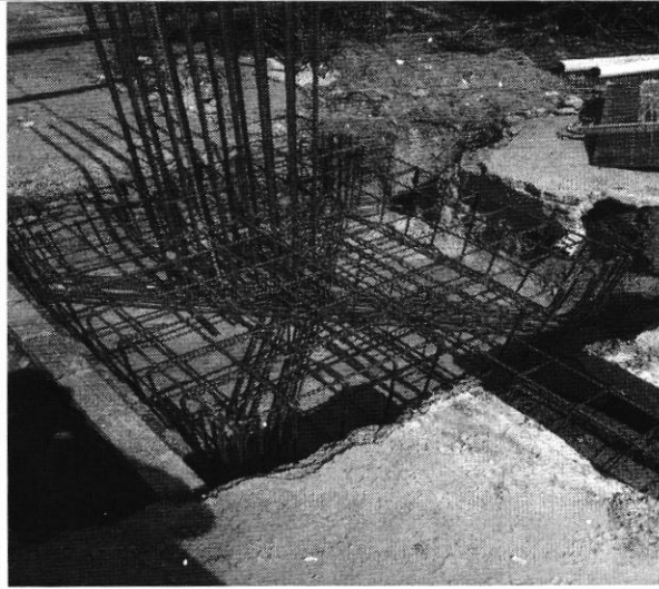
EXECUÇÃO BLOCOS DE FUNDAÇÃO DE ESTRUTURA DE CONCRETO
